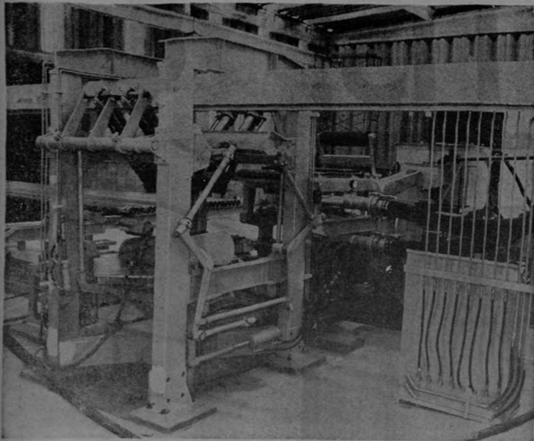
En esta fotografía puede apreciarse una de las máquinas instaladas en la nueva fábrica de tubos de asbesto-cemento RICALIT situada en Paraíso de Cartago, y que a fines de este año, estará en plena producción.
